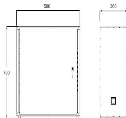
ARTICLE 7801 DIMENSIONS EN mm
