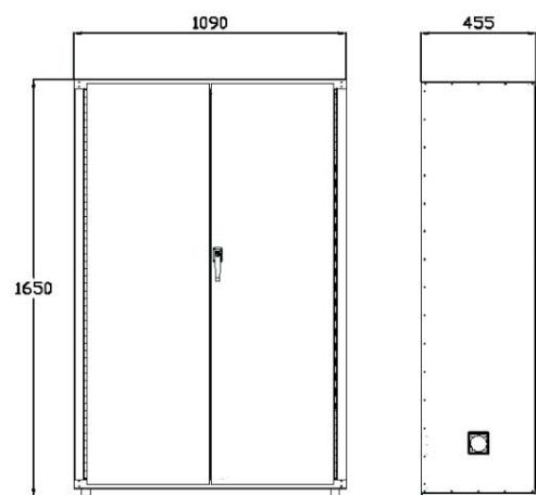
ARTICLE 7502 DIMENSIONS EN mm
