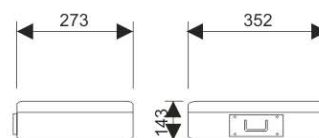
ARTICLE 7310 DIMENSIONS EN mm
