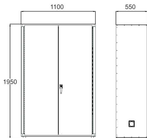
ARTICLE 7010BATA/30 DIMENSIONS EN mm
